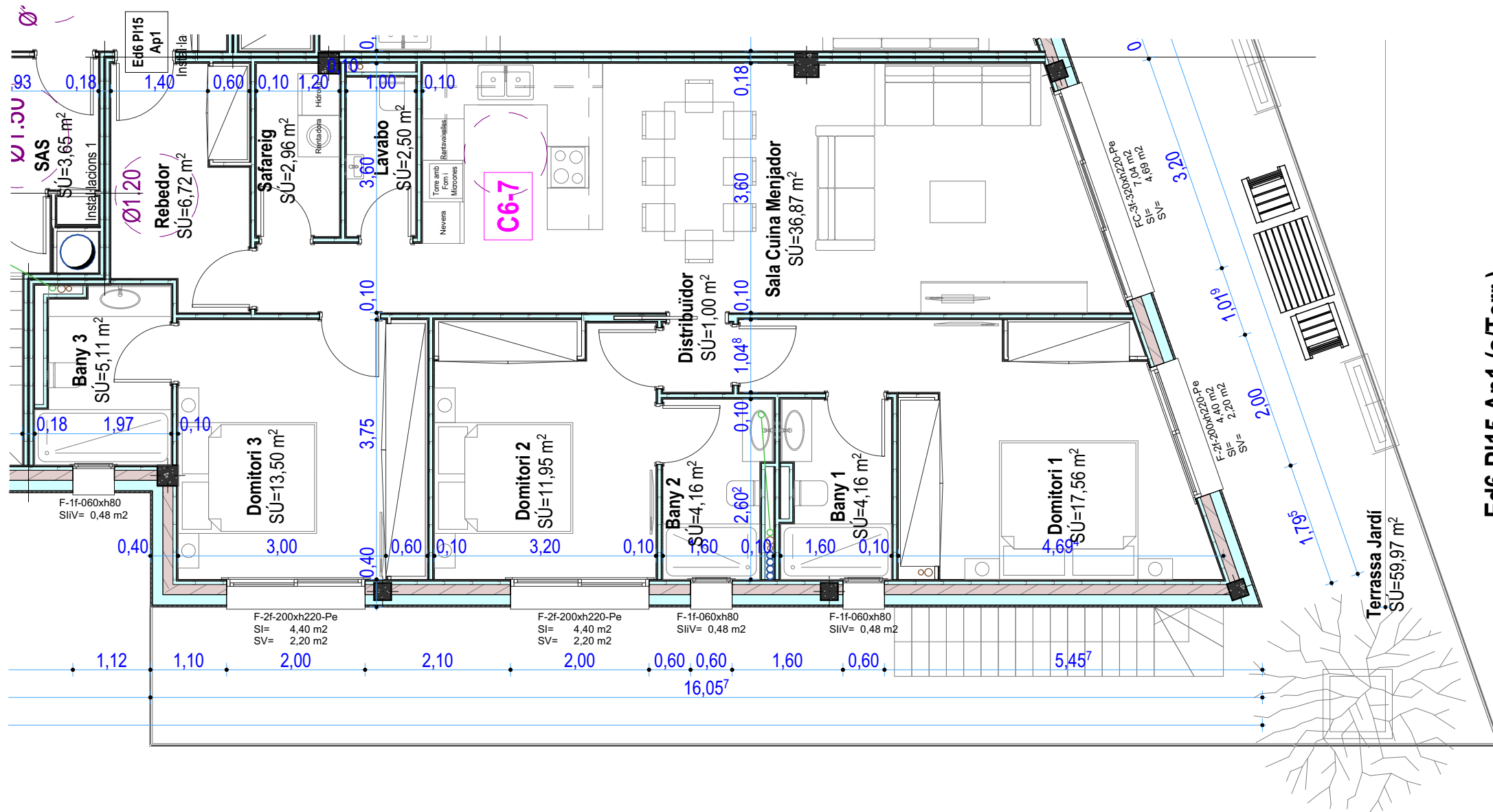
Planta Alta - Coberta Esc.: 1:150
